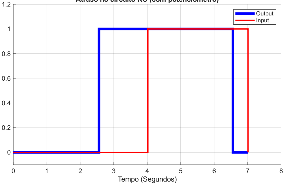
Atraso no circuito RC (com potenciômetro)
